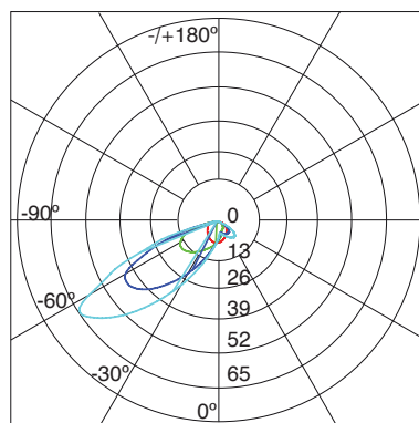
Distribución Polar Candelas / Polar distribution UNIT: cd
